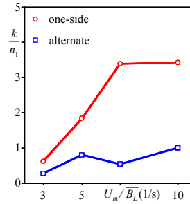
図-4 連続遡上挑戦率
