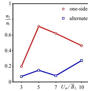
図-3 連続遡上率
