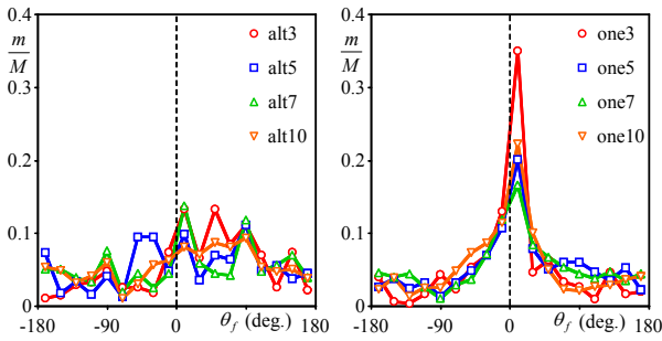
図-9 アユの魚向の頻度分布
