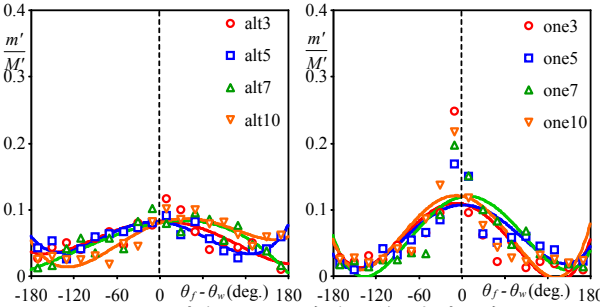
図-10 流向とアユの魚向の差の頻度分布
