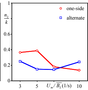
図-5 連続遡上成功率
