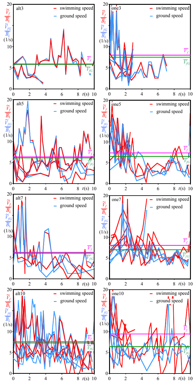
図-11 アユの対地速度および遊泳速度
