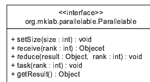
図 3: Parallelable インターフェース
