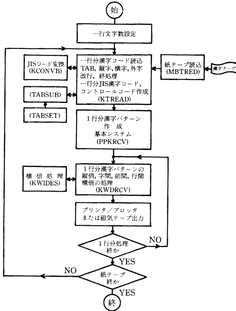
図-2 漢字コード紙テープ・コントロール処理の流れ
