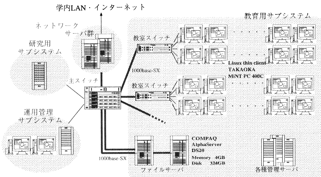
図 1: システム構成概要
