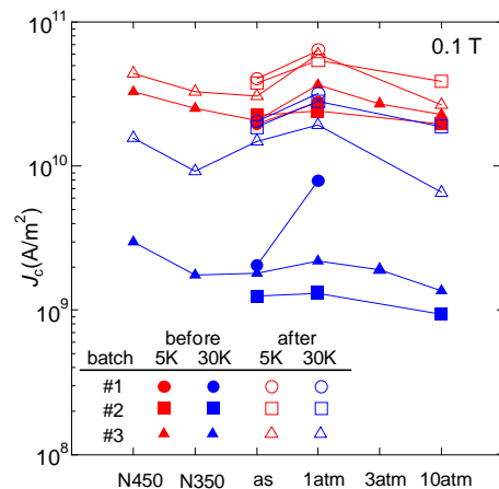
図4 さまざまなアニール条件における臨界電流密度の関係。
