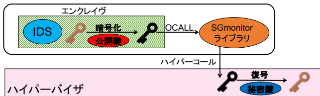
図 6 暗号鍵の共有
