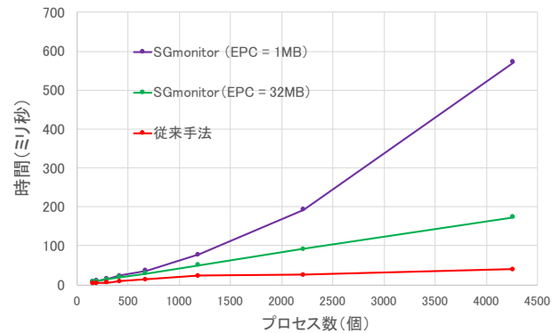
図 10 プロセス数と EPC サイズの影響
