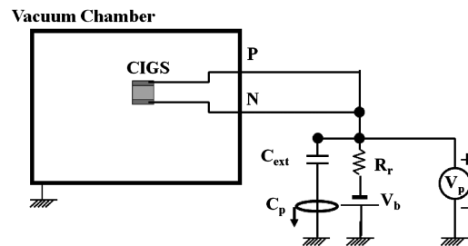
Fig. 4 Discharge circuit.
