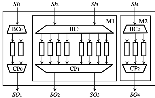
Fig. 9. Hierarchical VirtualScan
